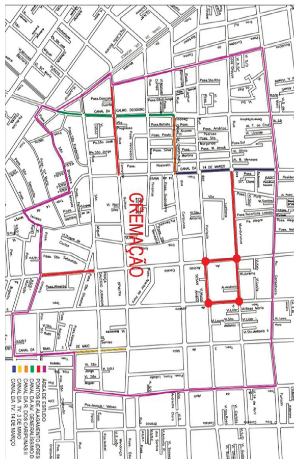
Figura 3. Canais de macrodrenagem estudados e localização dos pontos de armazenamento segundo DRES.
