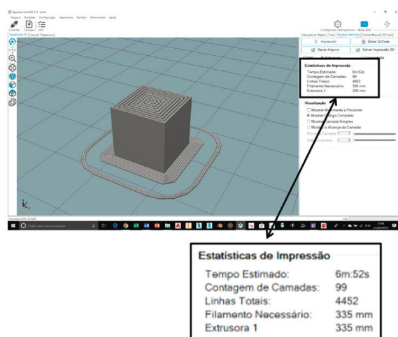
Figura 10. Especificações do programa de impressão 3D.
