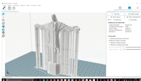
Figura 13. Modelo fatiado e com suportes.
