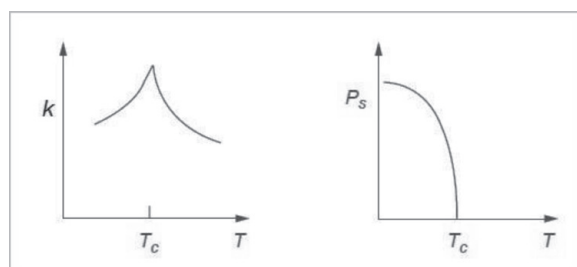
Figura 1 - Ilustração esquemática da constante dielétrica no eixo z ( \kappa ) e a polarização espontânea P_s com a temperatura, para o KDP.
