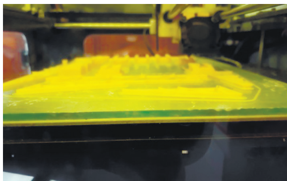
Figura 04. Início do processo de impressão com a bandeja na parte superior.
