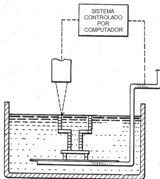
Figura 03. Ilustração do processo da primeira impressora 3D de Charles Hull.
