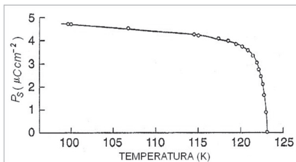
Figura 4- Polarização espontânea do cristal de KDP como uma função da temperatura.
